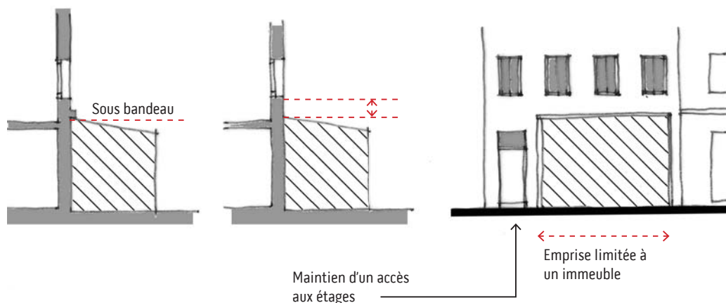
terrasse fermée sur le domaine public, principes d'implantation
