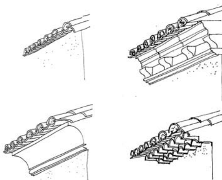
Débord de toits autorisés
